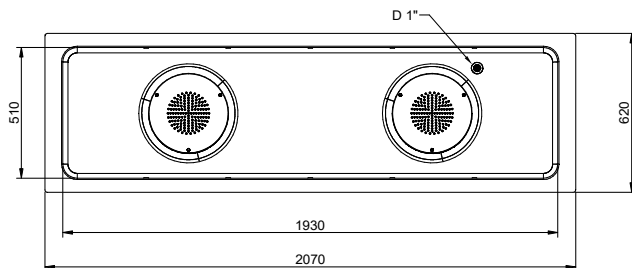
Boven aanzicht
